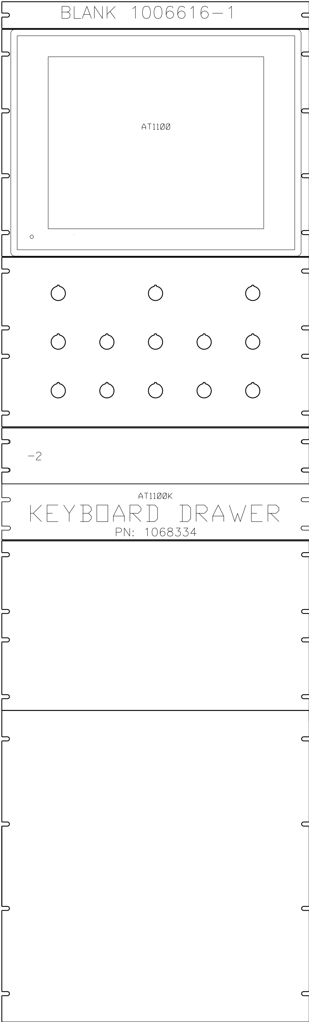
LEFT/FRONT
